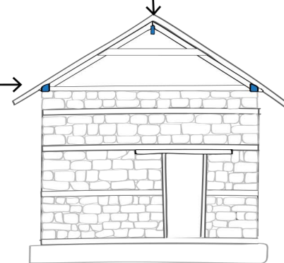
धुरी बलो र कैचीको जोडाई
