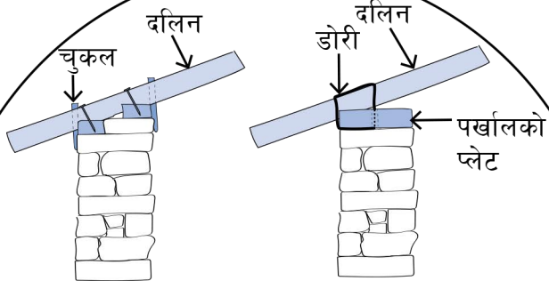
छाना र दलिनको जोडाई #१
